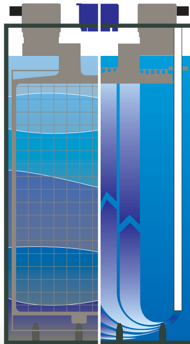
Elektrolytschichtung mit unterschiedlicher Dichte Elektrolytumwälzung nach dem AirLift-Prinzip
